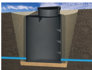
Vodoměrná šachta - ukázka uložení
